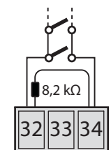
Parallel geschaltet bei resistiven Schaltleisten 8,2 k \Omega
