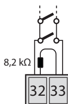
Parallel geschaltet bei resistiven Schaltleisten 8,2 k \Omega
